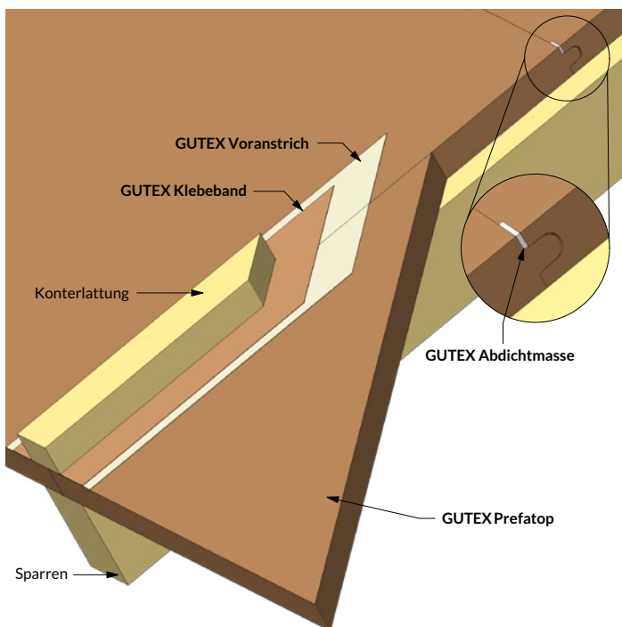
Stoßdetail/-abdichtung bei Dachelementen mit GUTEX Prefatop (Detail 1.1.601)
